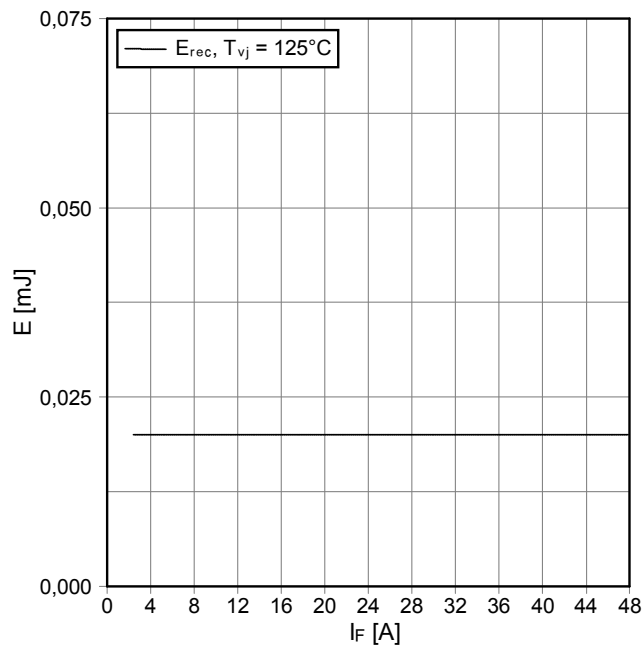
Schaltverluste Diode-Brems-Chopper (typisch) switching losses diode-brake-chopper (typical) E_{rec} = f(I_F) R_{Gon} = \Omega, V_{CE} = 300\text{ V}
