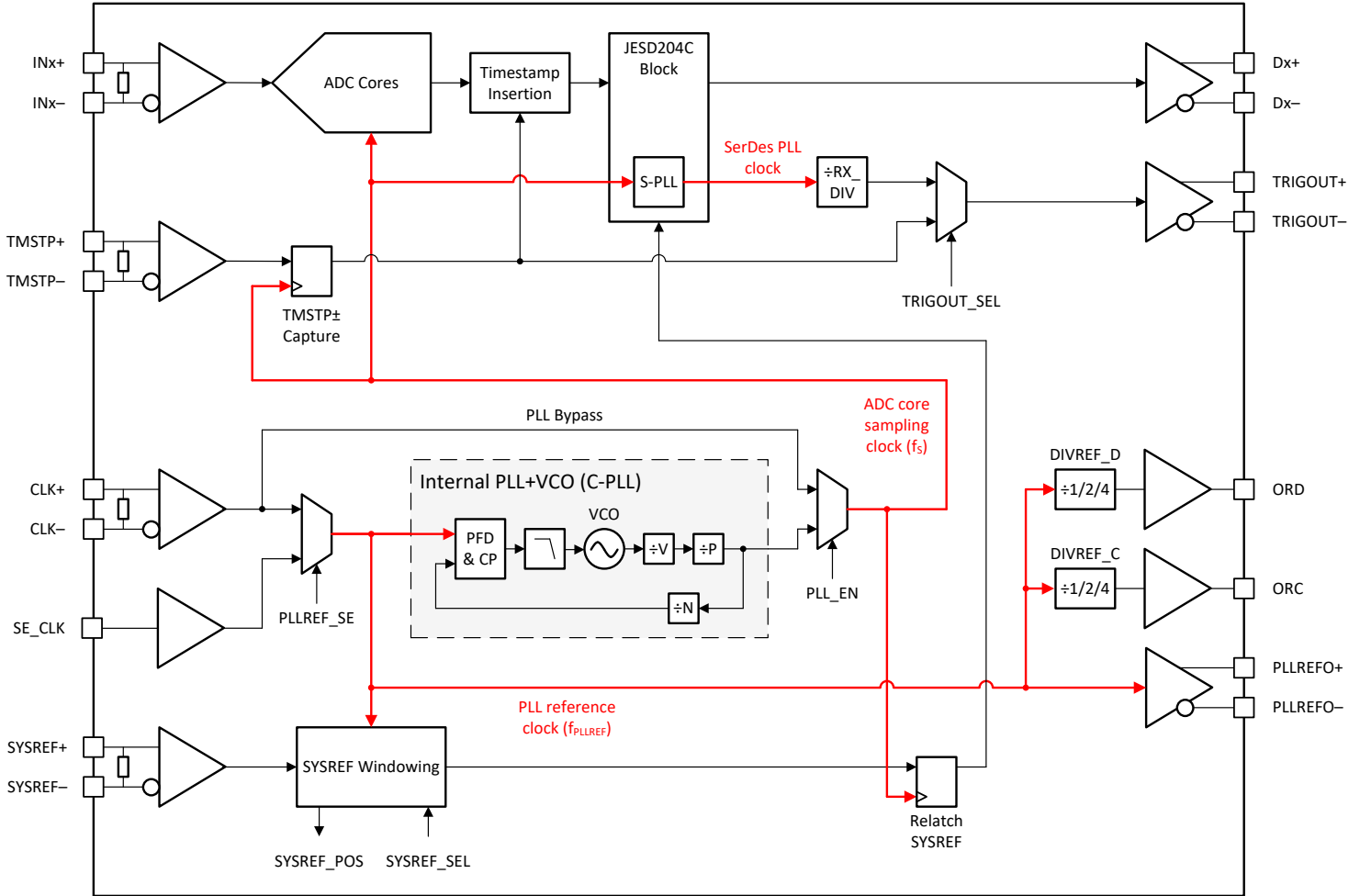
图 8-5. Clocking Subsystem
