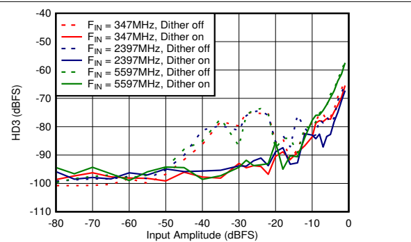
图 6-64. DES Mode: HD3 vs Input Amplitude and Dither
