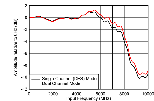
图 6-1. Input Amplitude vs Input Frequency
