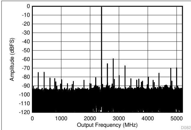
图 6-7. DES Mode: Single Tone FFT at 2397 MHz
