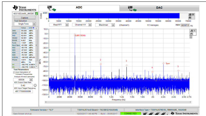
图 8-2. FFT for 497.77-MHz Input Signal, 5.4 GSPS, JMODE0
