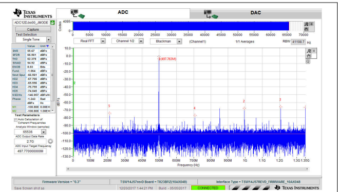
图 8-3. FFT for 497.77-MHz Input Signal, 2.7 GSPS, JMODE2
