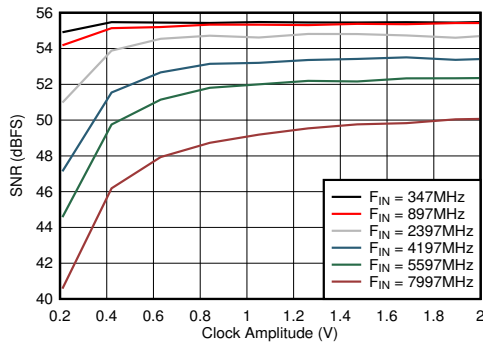
图 6-81. DES Mode: SNR vs Clock Amplitude
