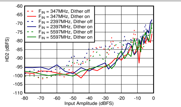
图 6-62. DES Mode: HD2 vs Input Amplitude and Dither
