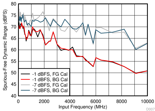
图 6-16. SFDR vs Input Frequency
