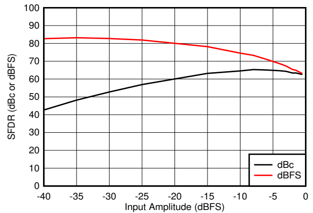
图 8-32. SFDR vs A_{IN}
