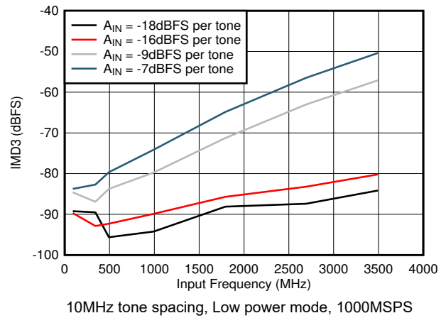
图 8-76. IMD3 vs F_{IN}
