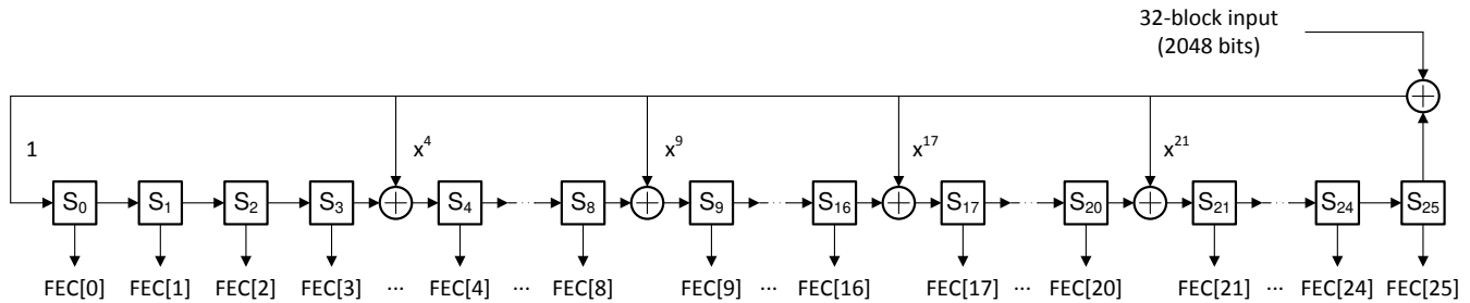
图 9-10. FEC Parity Bit Generator
