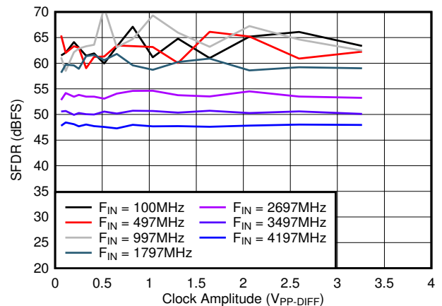
图 8-36. SFDR vs A_{CLK}
