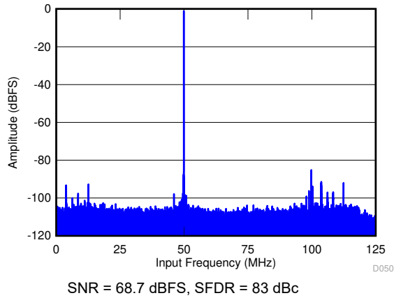
图 7-53. FFT for 450-MHz Input Signal in Decimate-by-4 Mode
