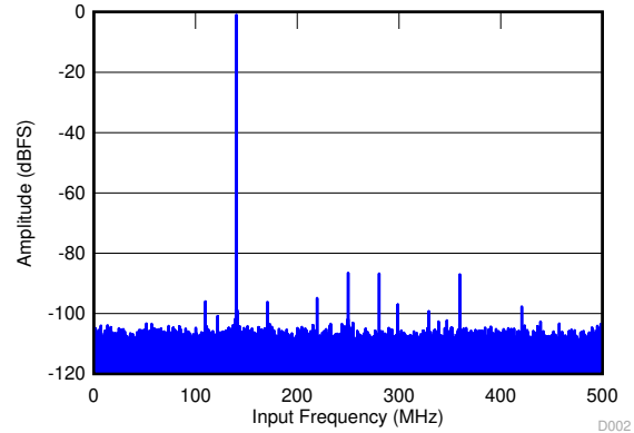
图 7-4. FFT for 140-MHz Input Signal
