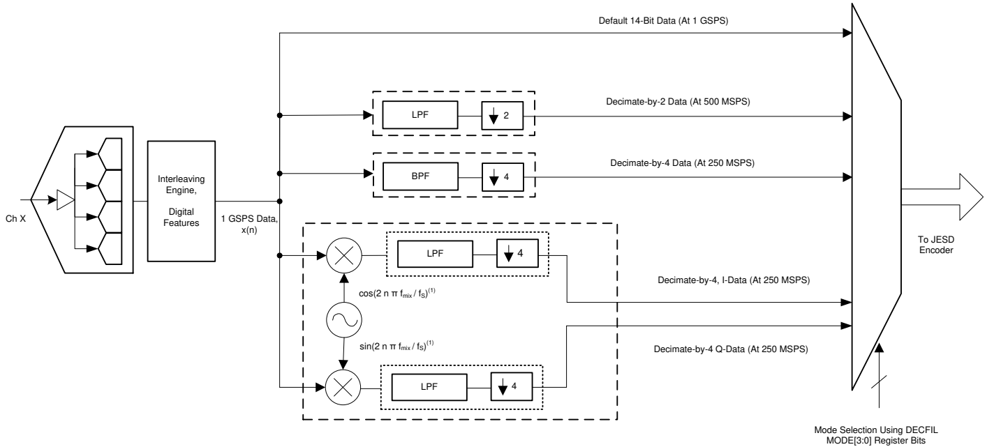
图 8-3. DDC Block
