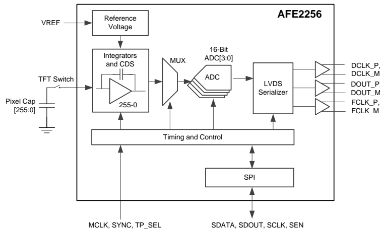
AFE2256 原理图
