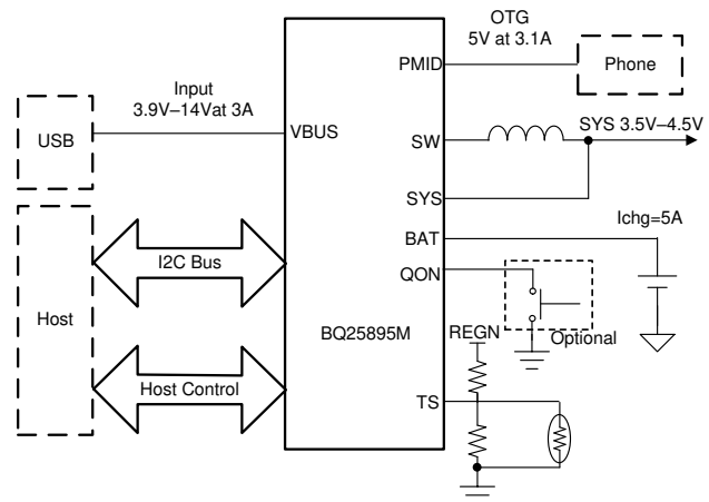
简化原理图
