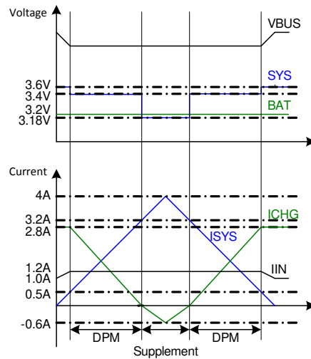
图 8-3. DPM Response
