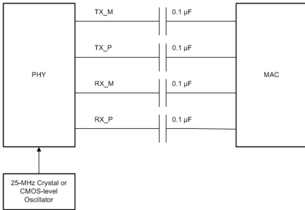
图 7-16. SGMII 连接
