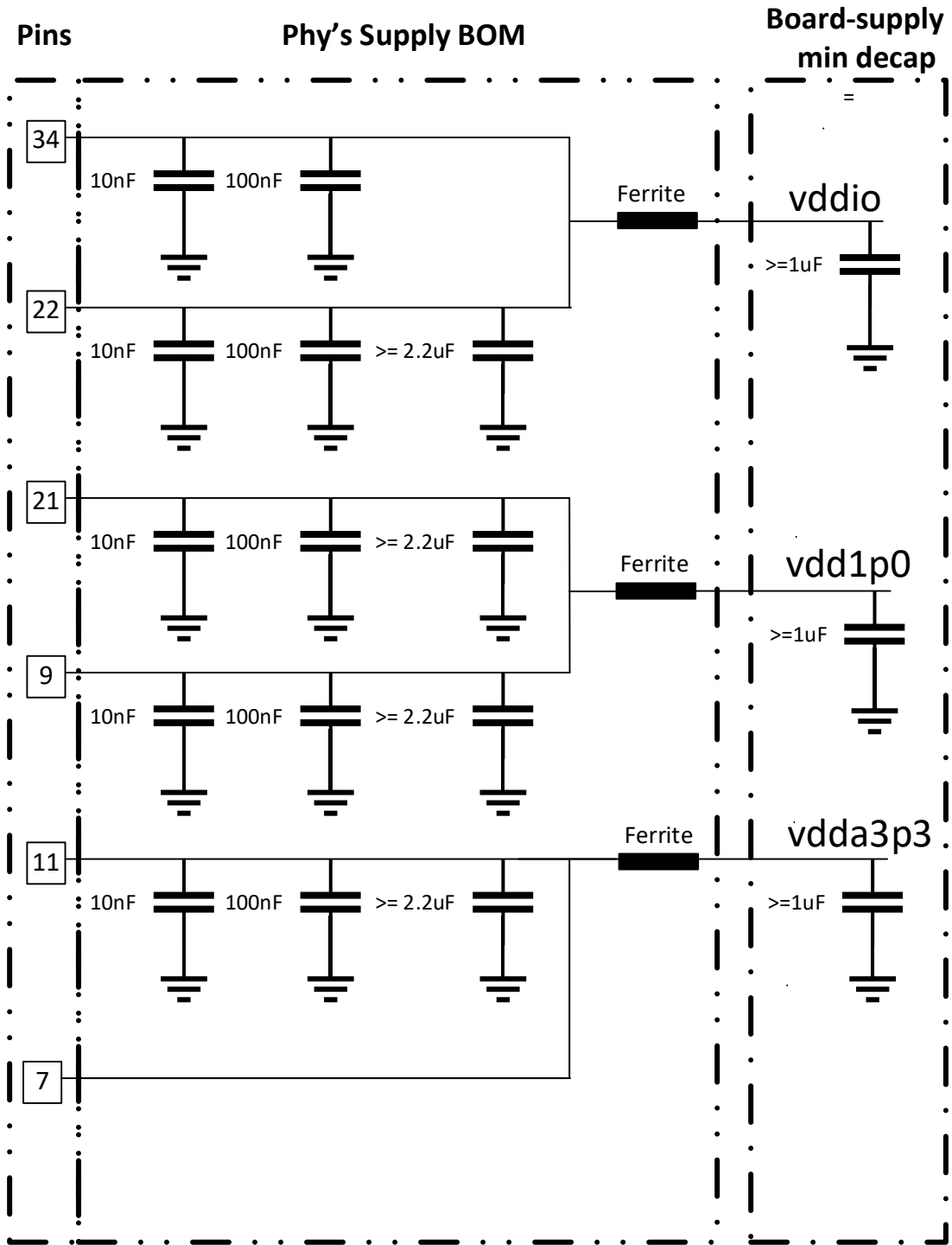
图 9-2. 建议电源去耦网络 (如果应用未采用睡眠模式)
