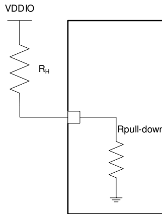
图 7-18. 设置电路
