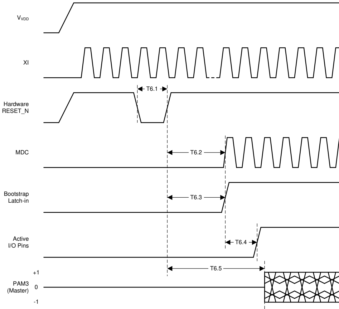
图 6-2. 复位时序
