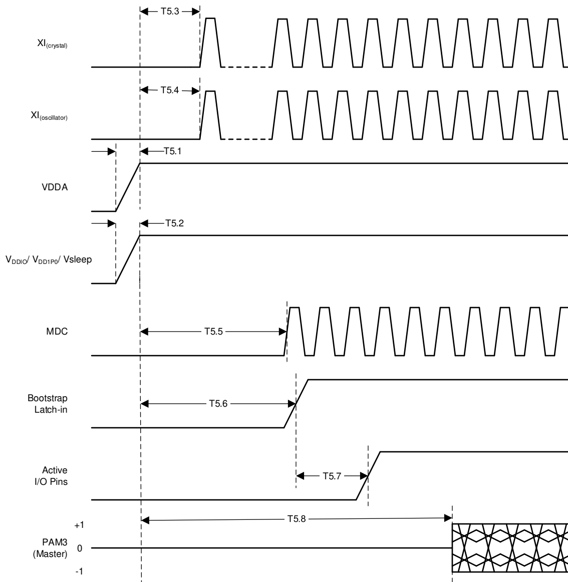
图 6-1. 上电时序
