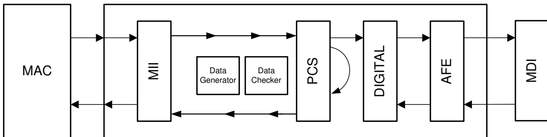
图 7-8. 具有外部数据生成器的 PCS 环回
