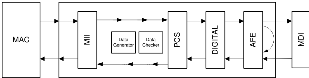
图 7-2. 所有环回
