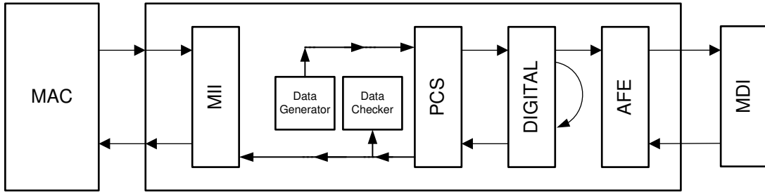
图 7-5. 具有内置数据生成器的数字环回
