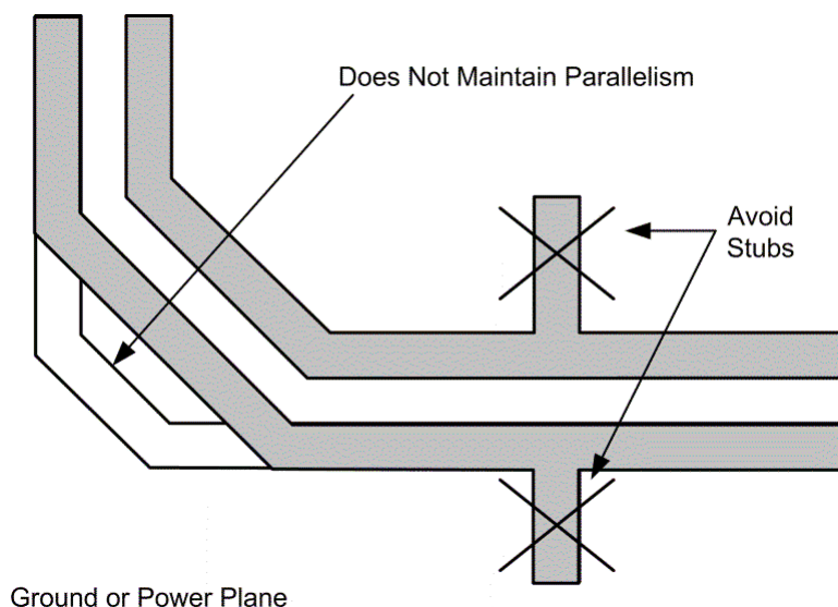
图 11-1. 差分信号布线
