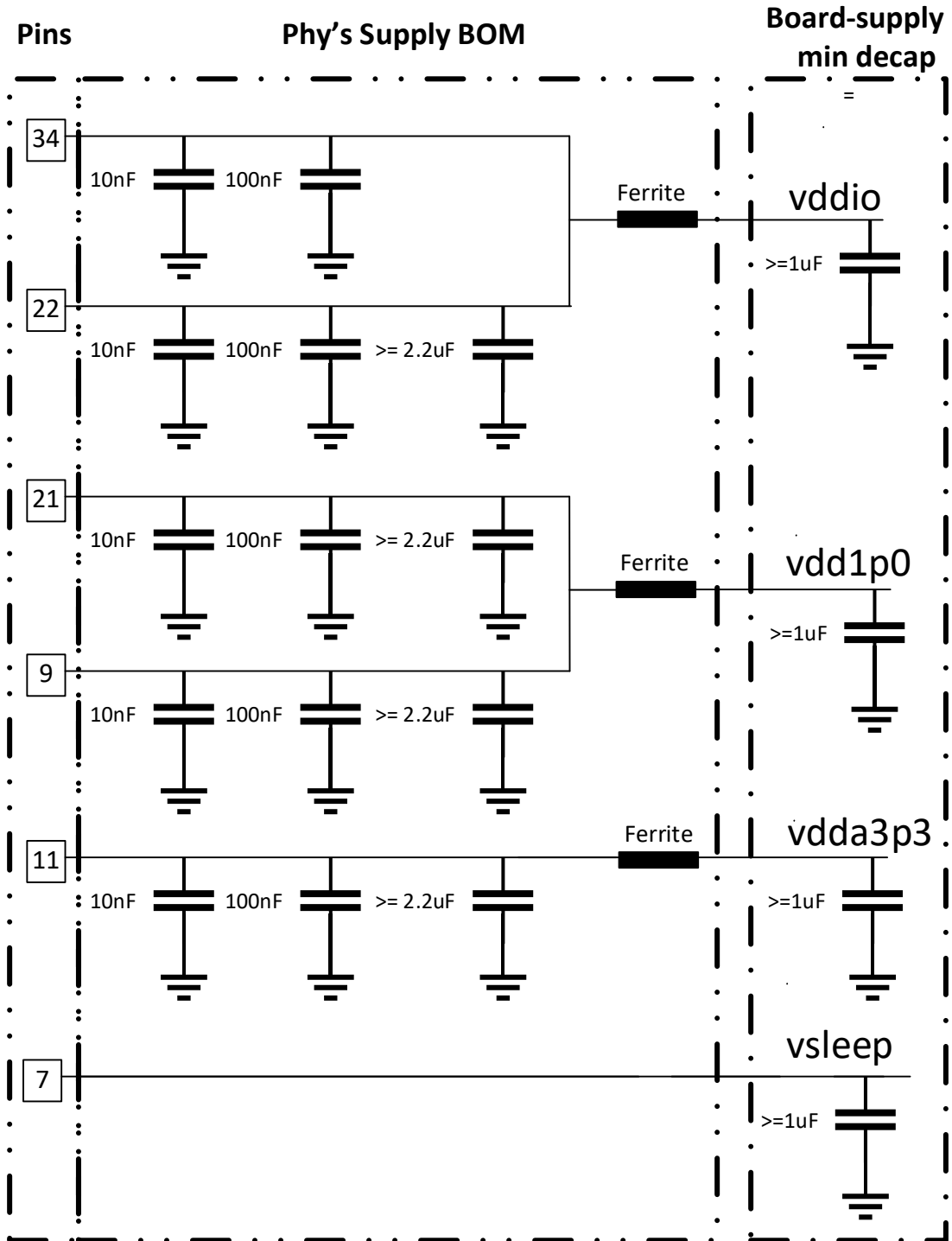
图 9-1. 建议电源去耦网络 ( 如果应用采用睡眠模式 )
