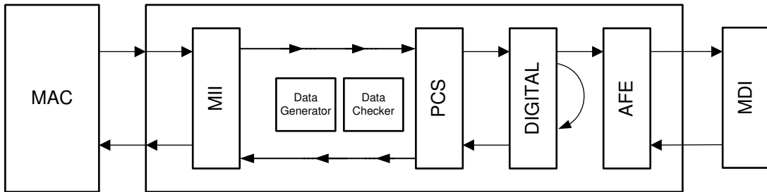
图 7-6. 具有外部数据生成器的数字环回
