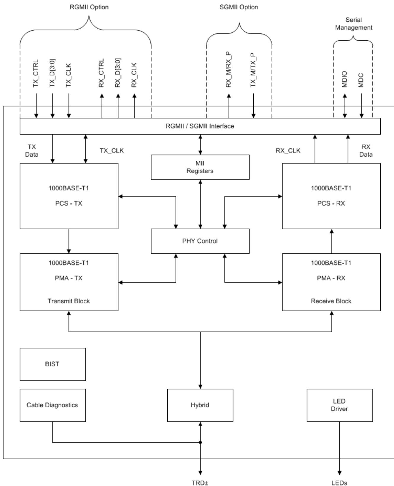
图 7-1. DP83TG720S-Q1 功能方框图
