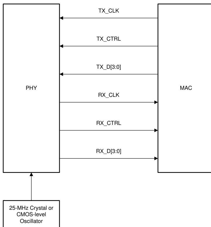
图 7-13. RGMII 连接
