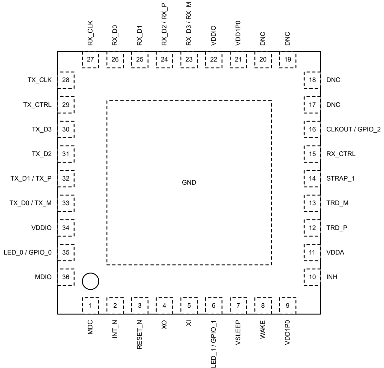
图 5-1. RHA 封装 36 引脚 VQFN 俯视图
