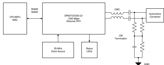
图 3-1. 简化原理图
