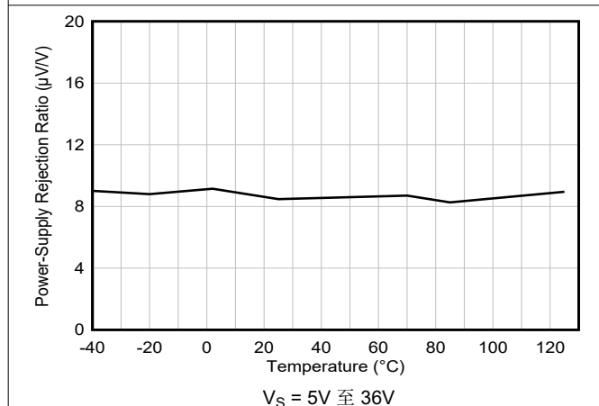
图 6-11. 电源抑制比与温度间的关系 V_S = 5\text{V} 至 36\text{V}
