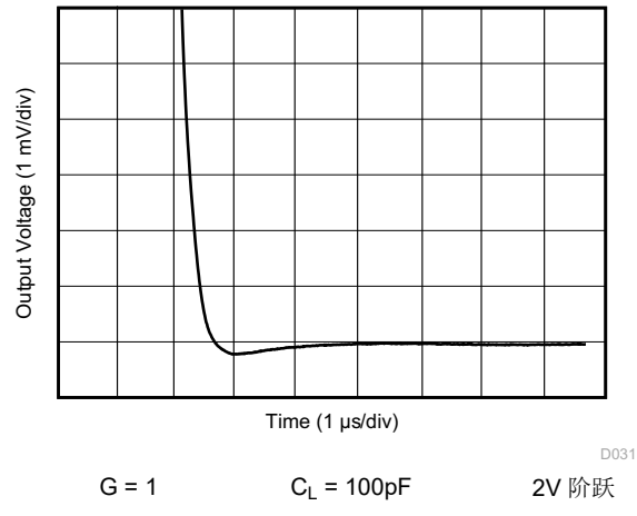
图 6-25. 大信号稳定时间 (负)
