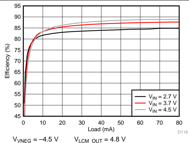
图 130. VNEG Efficiency
