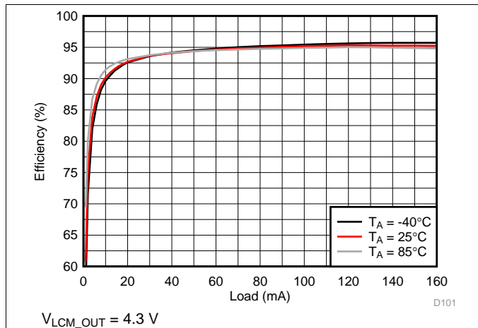
图 115. LCM Boost Efficiency
