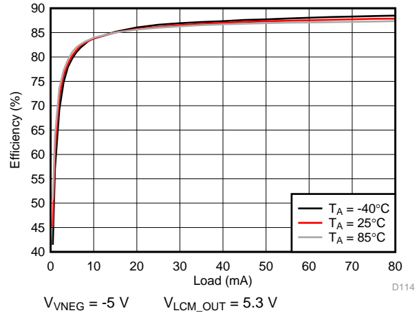
图 128. VNEG Efficiency
