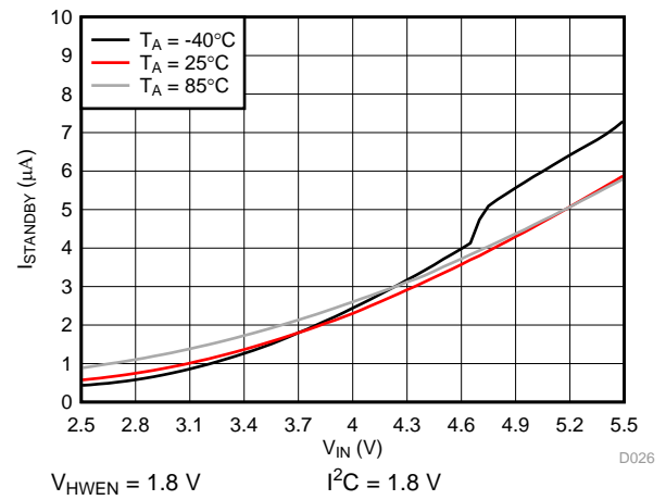
图 29. I_q Standby
