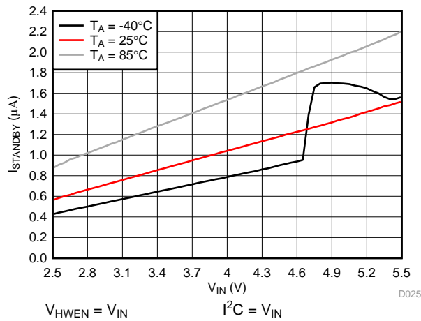
图 28. I_q Standby
