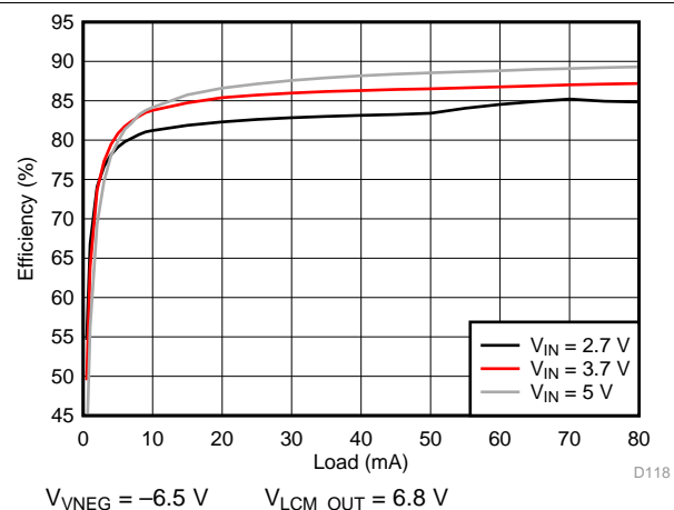
图 132. VNEG Efficiency
