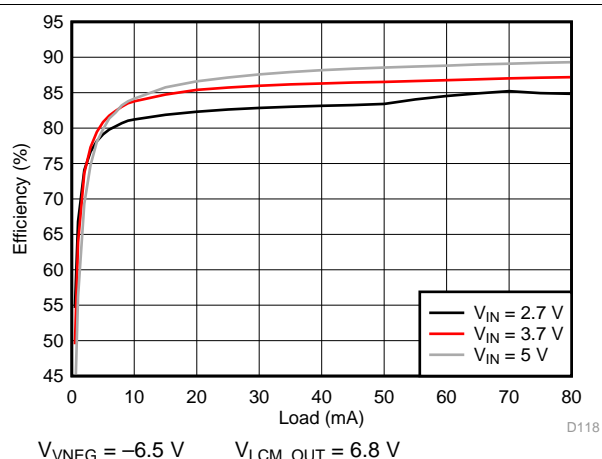
图 204. VNEG Efficiency
