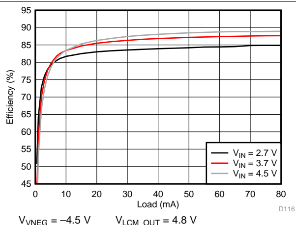
图 202. VNEG Efficiency
