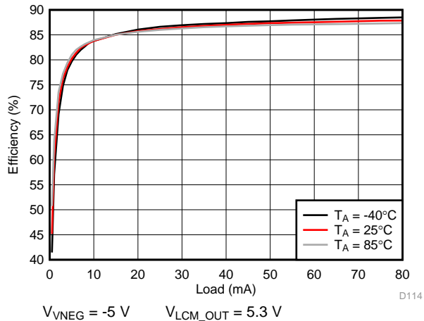
图 200. VNEG Efficiency
