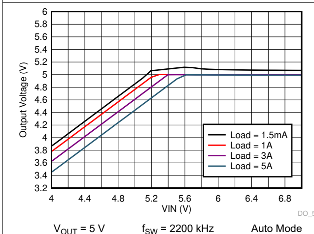
图 9-37. LM73605-Q1 Dropout Curve
