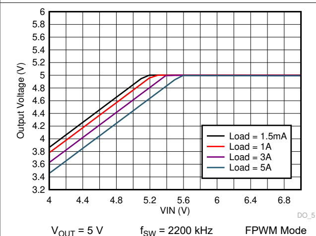
图 9-38. LM73605-Q1 Dropout Curve
