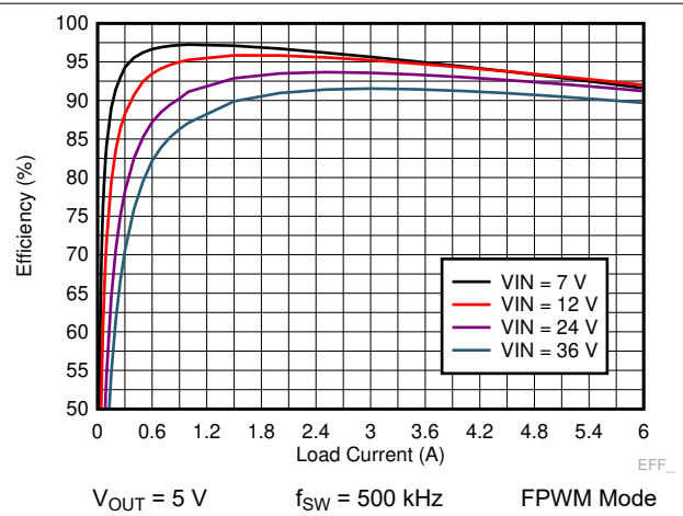
图 9-14. LM73606-Q1 Efficiency
