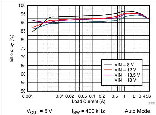
图 9-11. LM73606-Q1 Efficiency
