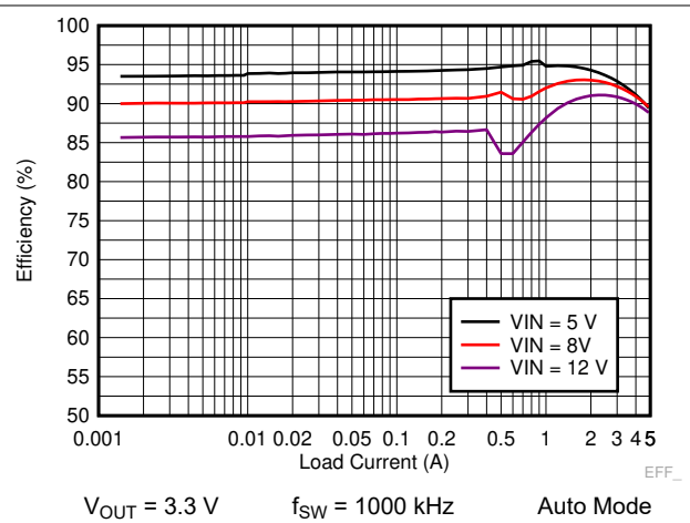
图 9-10. LM73605-Q1 Efficiency
