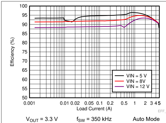
图 9-9. LM73605-Q1 Efficiency
