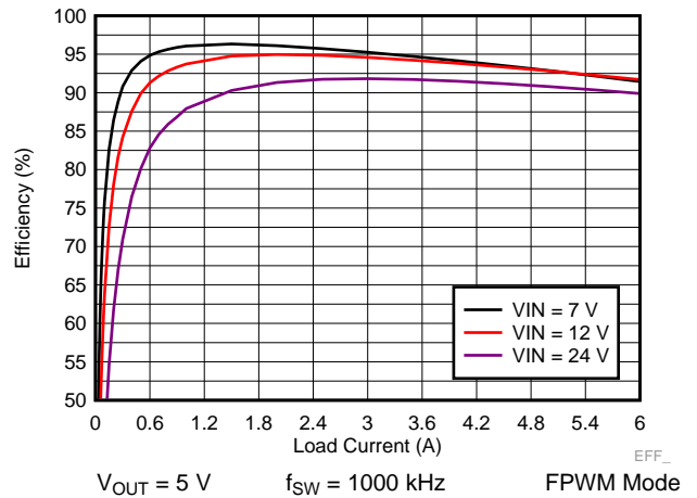
图 36. LM73606 Efficiency
