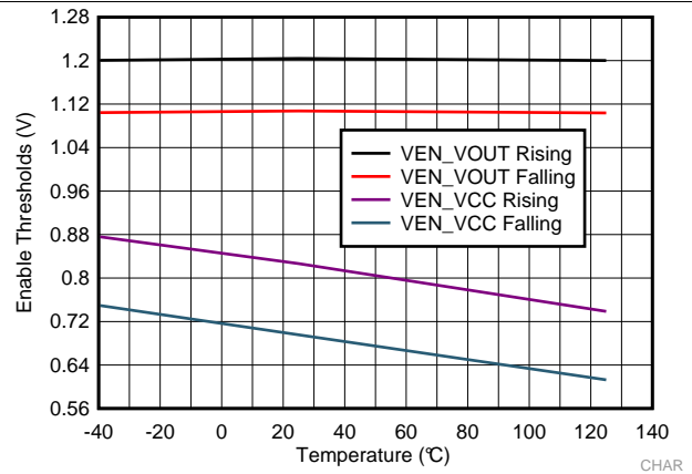
图 8. Enable Thresholds
