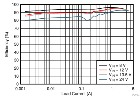
效率与输出电流 ( V_{\text{OUT}} = 5\text{V} , f_{\text{sw}} = 400\text{kHz} , 自动模式)
