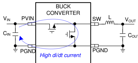
图 89. Buck Converter High di / dt Path
