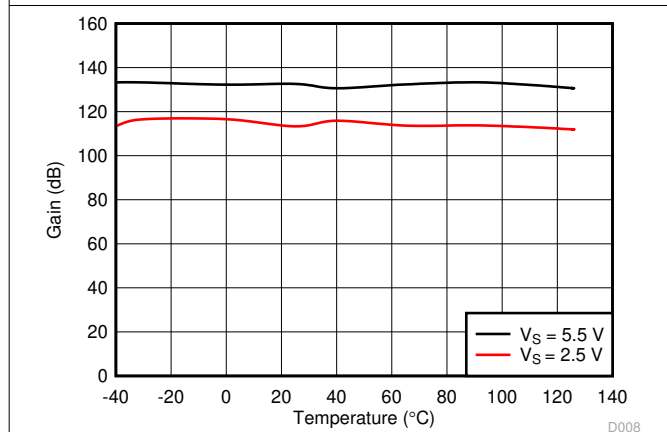
图 6-3. 开环增益与温度间的关系
