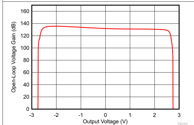
图 6-5. 开环增益与输出电压间的关系
