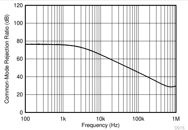
图 6-10. CMRR 与频率之间的关系
