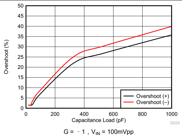
图 6-20. 小信号过冲与容性负载间的关系
