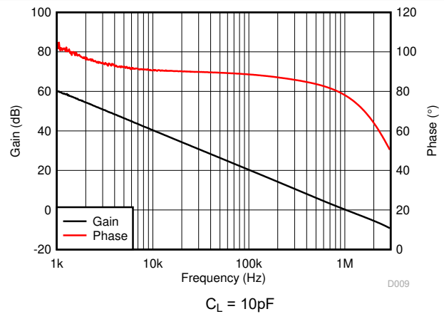
图 6-4. 开环增益和相位与频率间的关系
