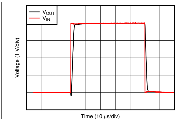
图 6-25. 大信号阶跃响应
