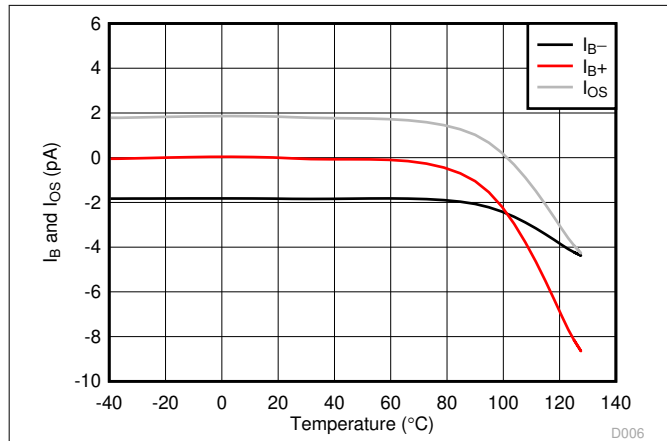
图 6-1. I_B 和 I_{OS} 与温度间的关系
