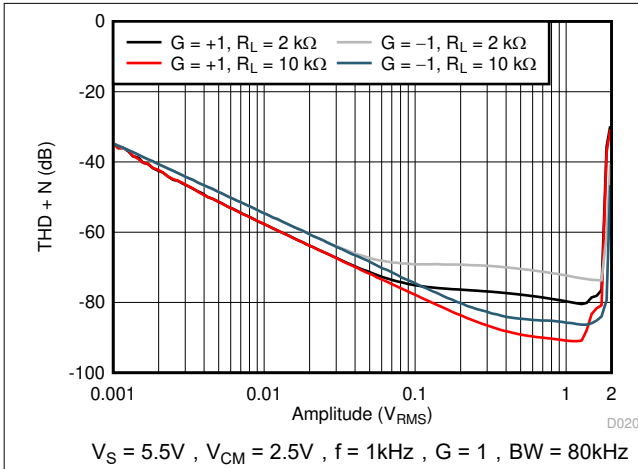
图 6-15. THD + N 与幅度间的关系
