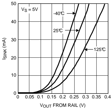
图 15. 灌电流与输出电压间的关系 (LMV651)
