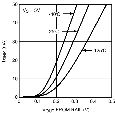
图 17. 灌电流与输出电压间的关系 (LMV654)
