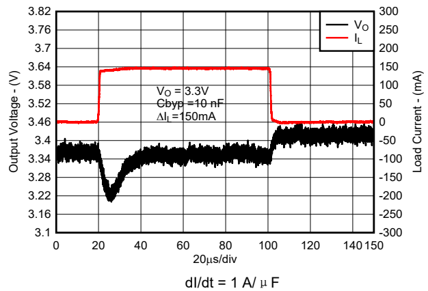
图 8-10. Load Transient for New Chip
