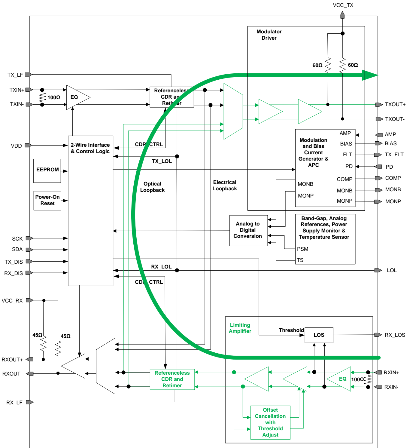
图 39. Optical Loopback
