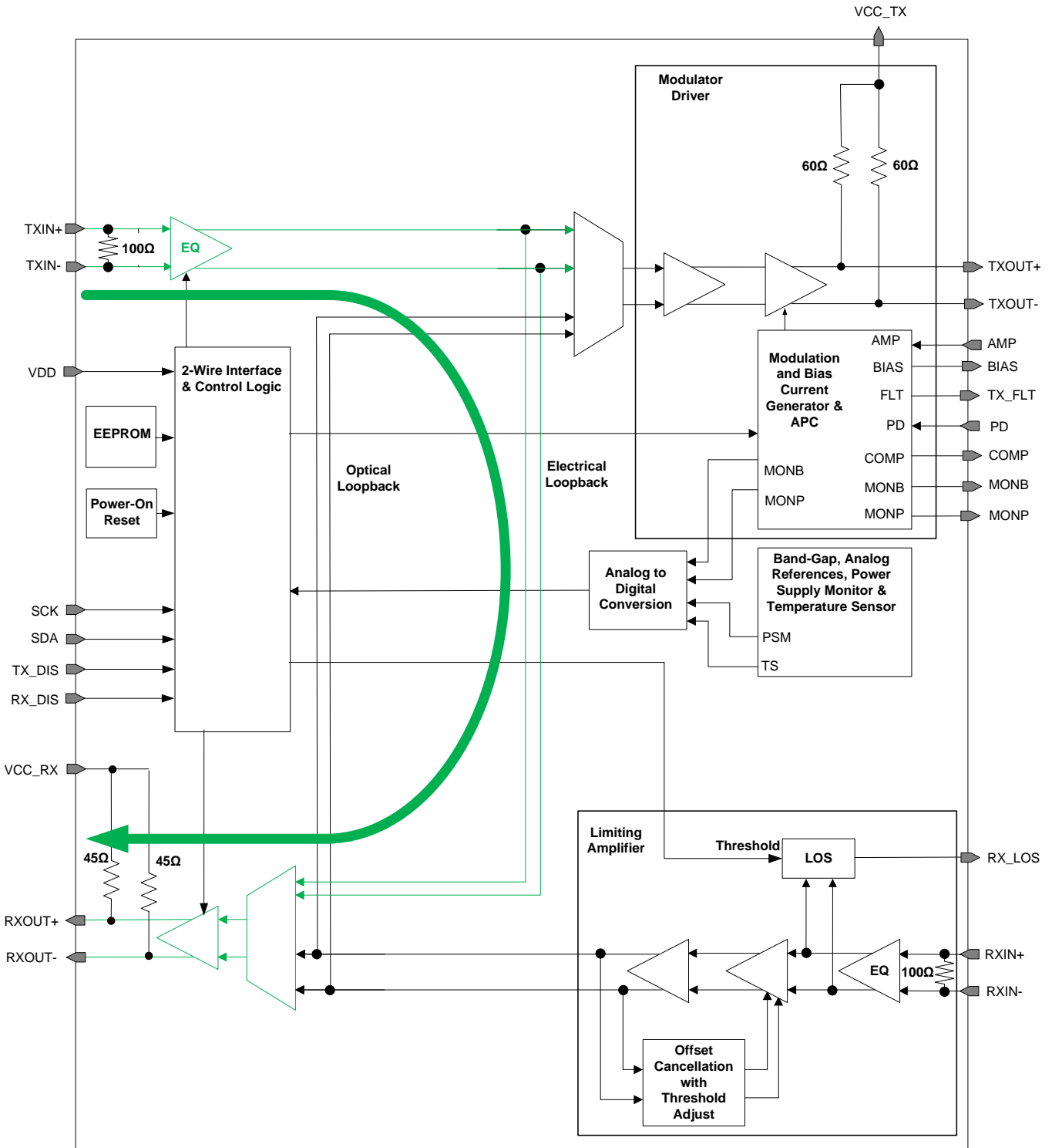
图 35. Electrical Loopback
