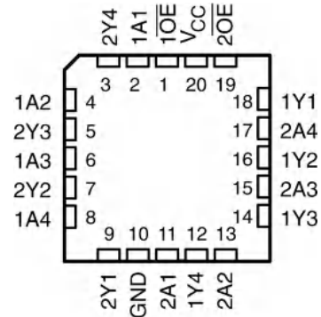
图 5-2. SN54AC240 FK Package (Top View)
