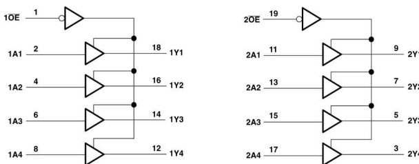
图 2-1. 逻辑图 (正逻辑)
