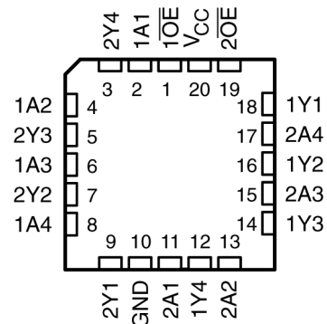
图 4-2. SN54AC244 FK Package (Top View)
