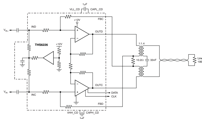
利用 THS6226 的一个端口的典型 VDSL2 线路驱动器电路
