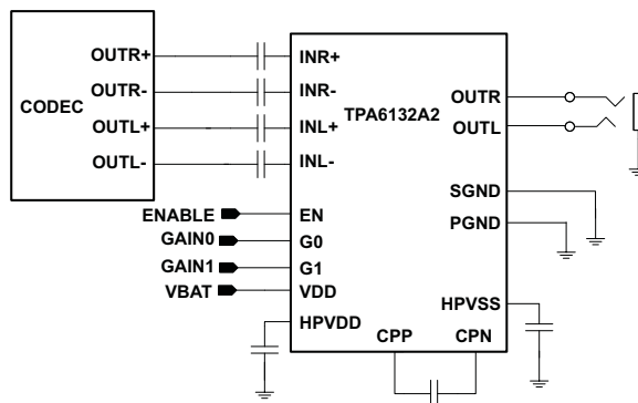
简化原理图
