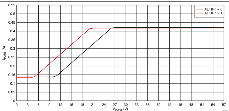
图 113. 浪涌折返曲线, I PORT 与 V PORT 间的关系
