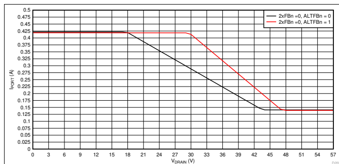
图 111. 1x 模式 (2xFBn = 0) 折返曲线, I PORT 与 V DRAIN 间的关系
