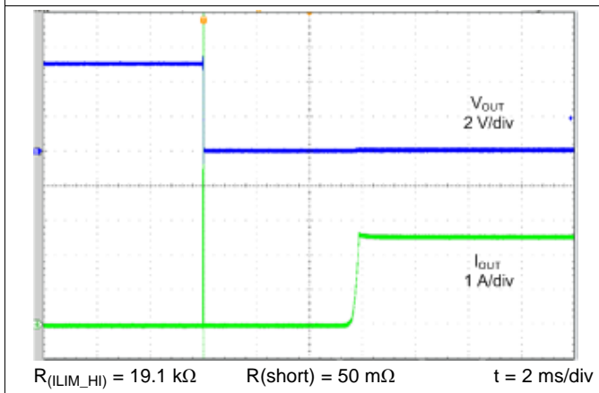
图 24. Hot Short
