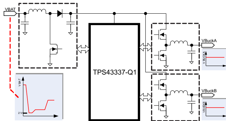
图 1. 典型应用图
