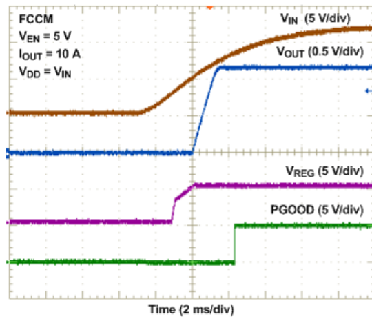
图 9-5. UVLO Start-Up
