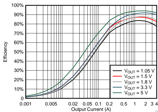
TPS564208 效率
