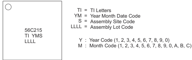
图 12-1. Symbolization
