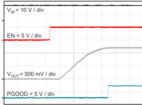
图 8-15. Start Up Relative to EN Rising
