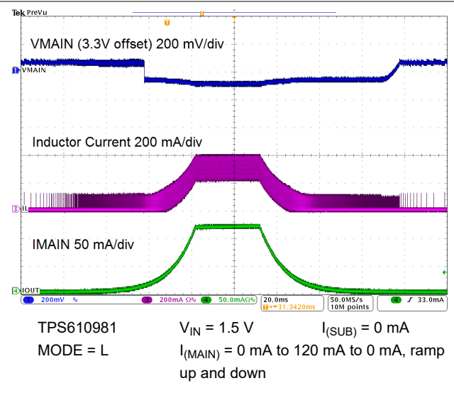
图 9-18. Load Regulation
