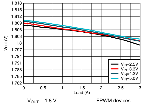
图 9-18. Load Regulation
