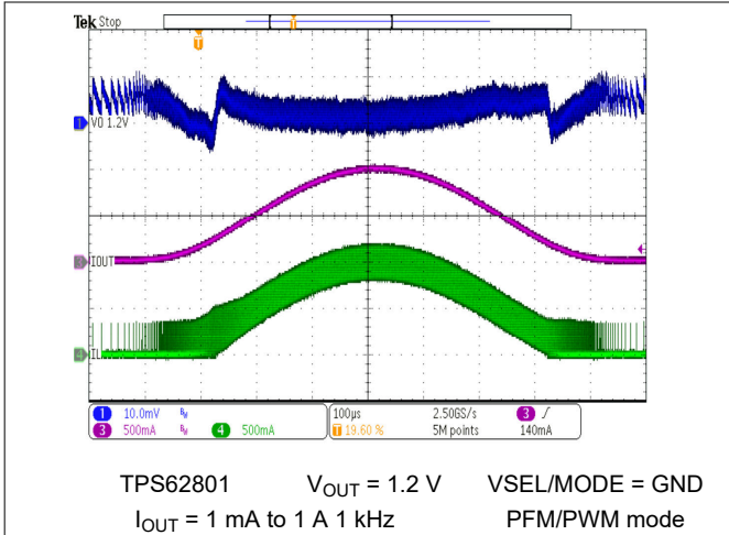
图 9-34. AC Load Sweep Power Save Mode
