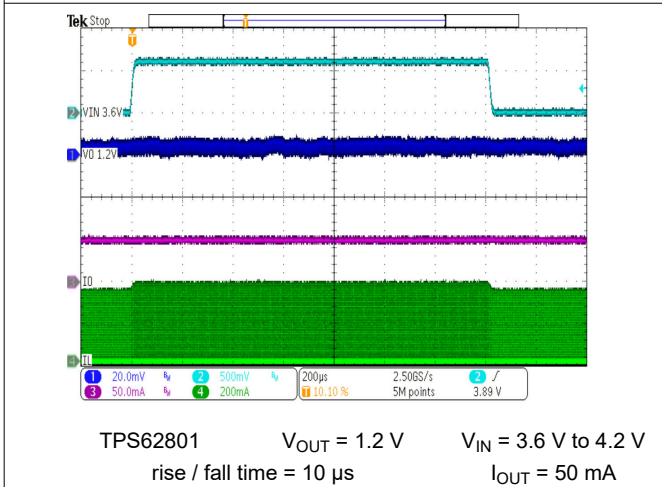
图 9-36. Line Transient PFM Mode
