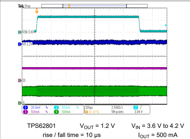
图 9-37. Line Transient PWM Mode
