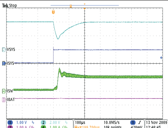
0-A - 1-A Transient on V_{SYS} V_{BUS} = 5.5\text{ V} No Battery V_{OREG} = 4\text{ V} I_{CHARGE} = 950\text{ mA} I_{IN\_limit} = 975\text{ mA}
