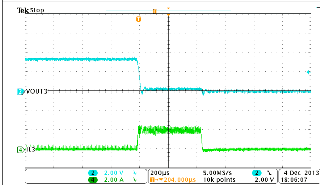
图 9-24. Buck3, OCP
