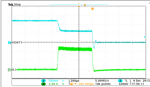
图 9-20. Buck1, OCP
