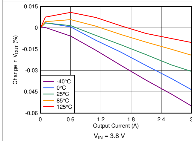
图 6-27. Load Regulation (3.3-V Output)
