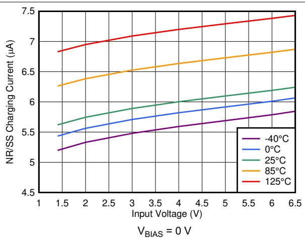
图 6-36. INR/SS Current vs Input Voltage
