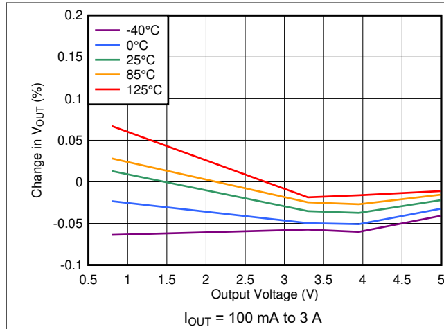
图 6-25. Load Regulation vs Output Voltage
