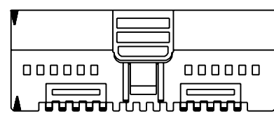
36 CKT. 18 CKT. DUAL ROW - EVEN
