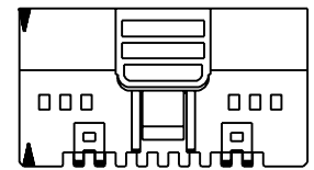
24 CKT. 12 CKT. DUAL ROW - EVEN
