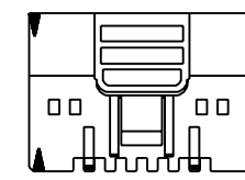
18 CKT. 9 CKT. DUAL ROW - ODD
